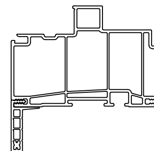
1" FLUSH FIN
